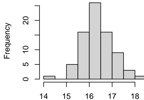
Ribose
